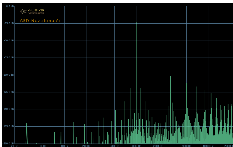
A5D-NAi THD (@ 0dBVU)
