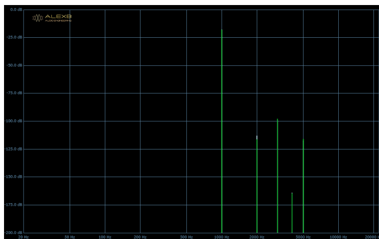
A5M-N·Ai THD (@ 0dBVU)
