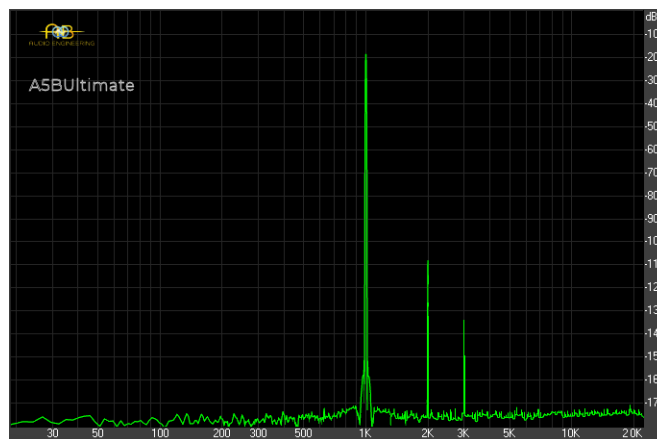
A5B THD (@ 0dBVU)
