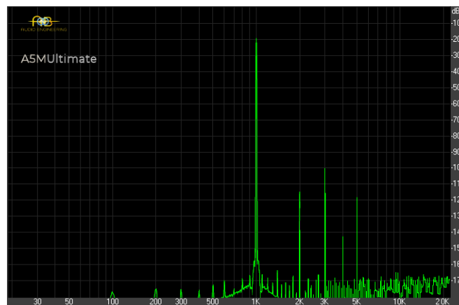
A5M THD (@ 0dBVU)
