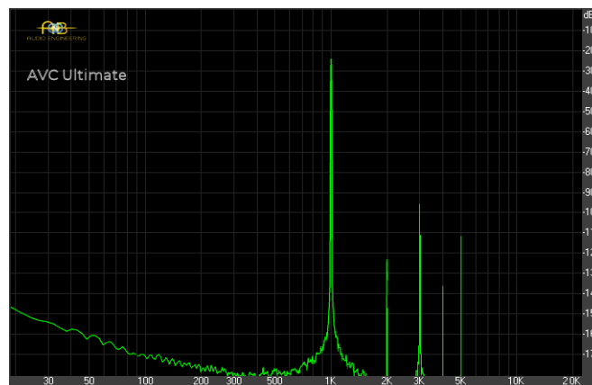
AVC THD (@ 0dBVU)
